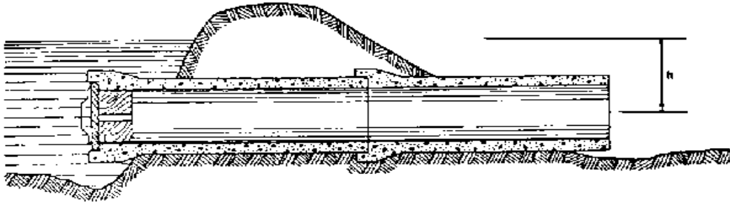
Fig. 2.13 (A pipe turnout)
