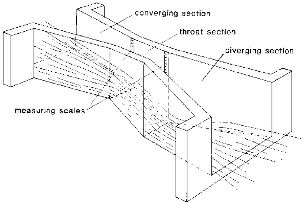
Fig. 3.2 (A Parshall flume)
